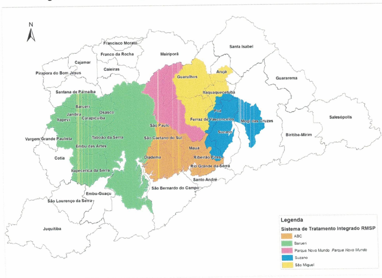
Figura 22 - Sistema Integrado de Esgotamento Sanitário da RMSP
