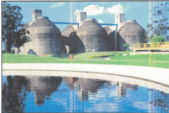
Figura 33 - Decantador Secundário e Digestores
