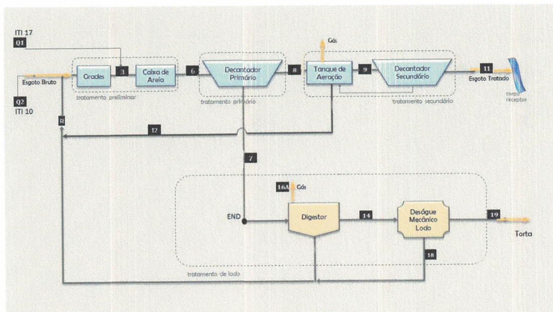
Figura 25 - Fluxograma simplificado do processo da ETE Suzano
