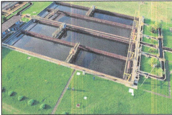
Figura 31 - Decantador primário
