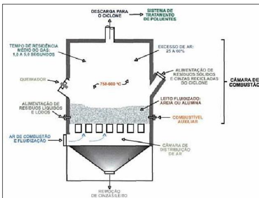
Figura 56 - Esquema de incinerador de leito fluidizado.
