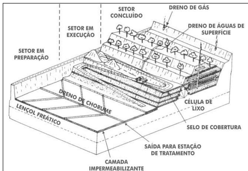
Figura 71 – Projeto técnico de aterro sanitário.
