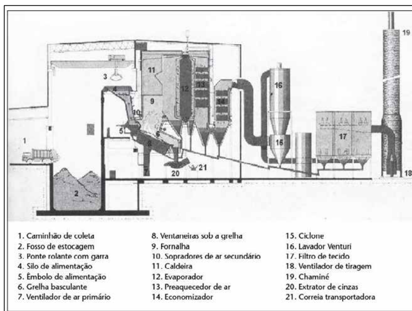
Figura 53 - Esquema de Incinerador de grelhas.
