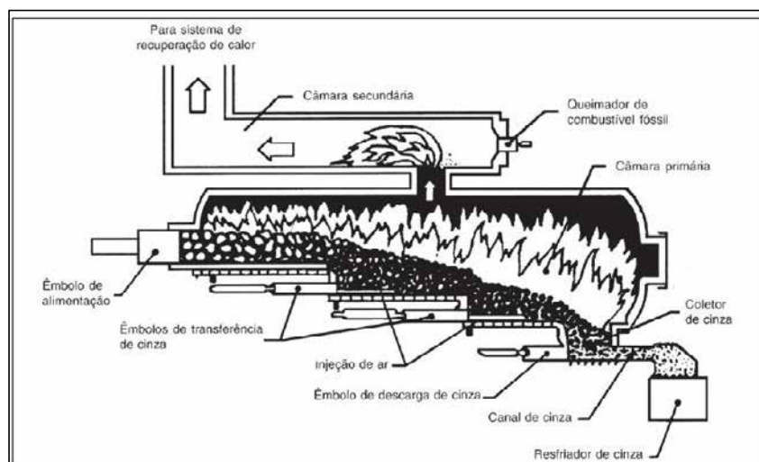
Figura 55 - Exemplo de incinerador em câmaras.
