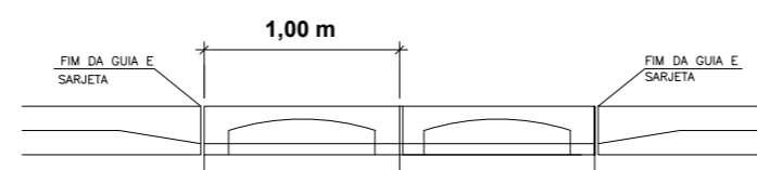
ELEVAÇÃO
