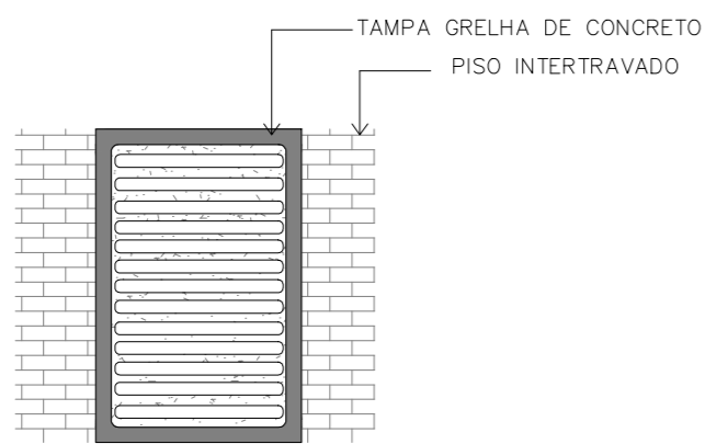
PLANTA
