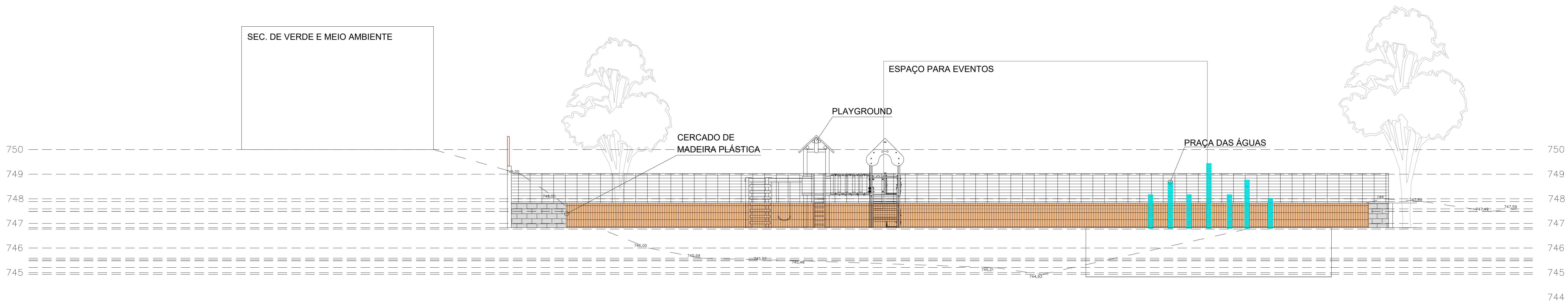
CORTE AA – PLAYGROUND/COTA DE IMPLANTAÇÃO 746,83 ESCALA 1/75
