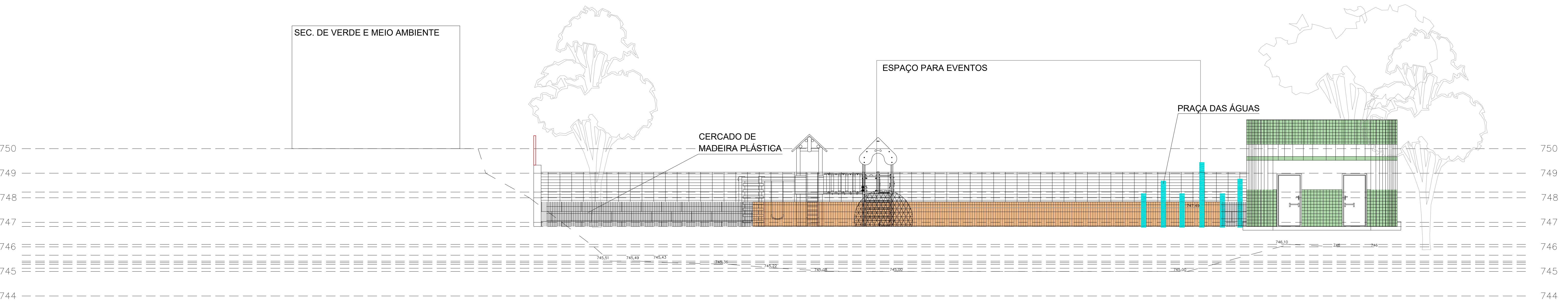
CORTE BB – PLAYGROUND/COTA DE IMPLANTAÇÃO 746,83 ESCALA 1/75
