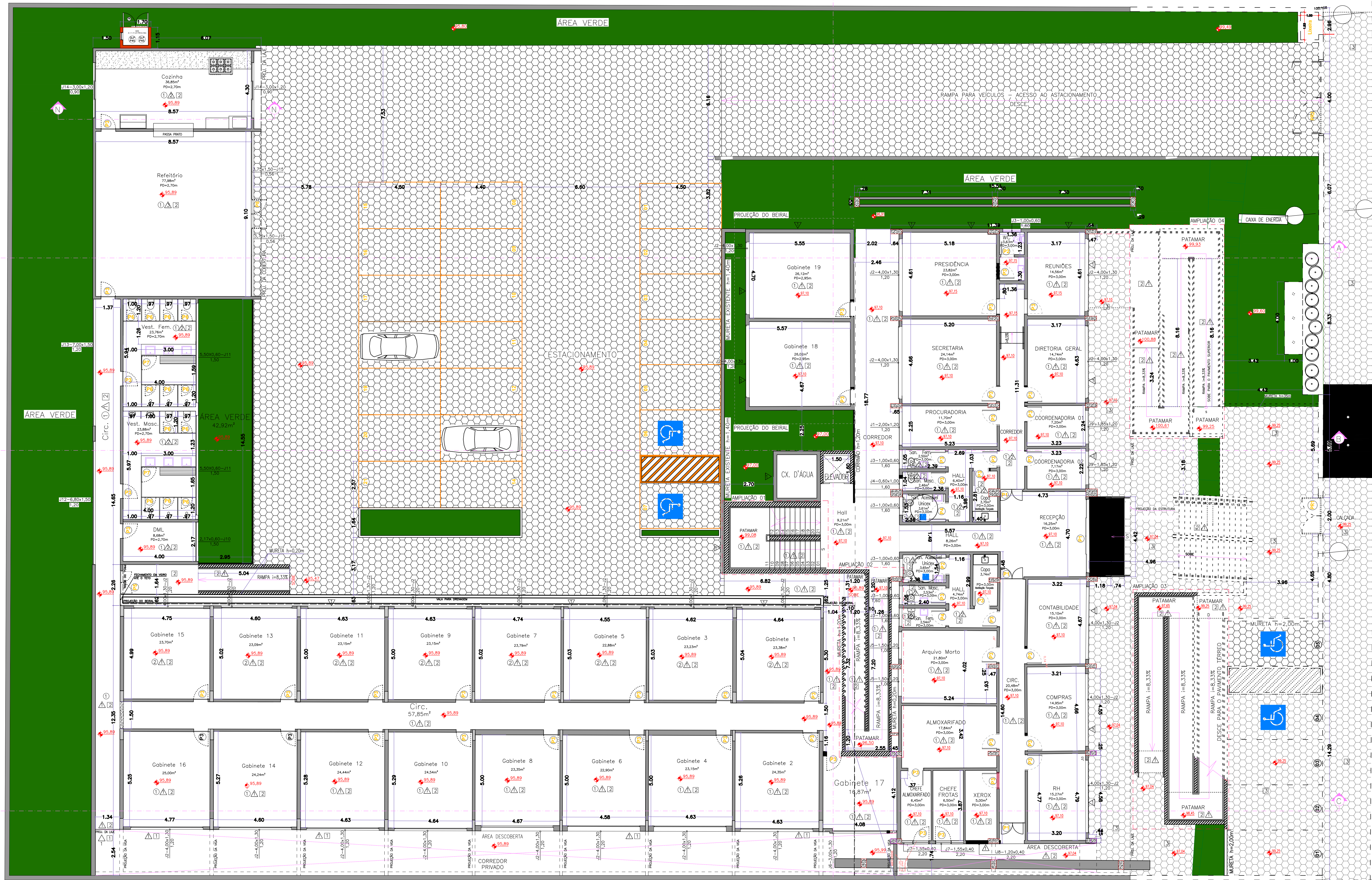
PLANTA PAV. TERREO escala 1:100
