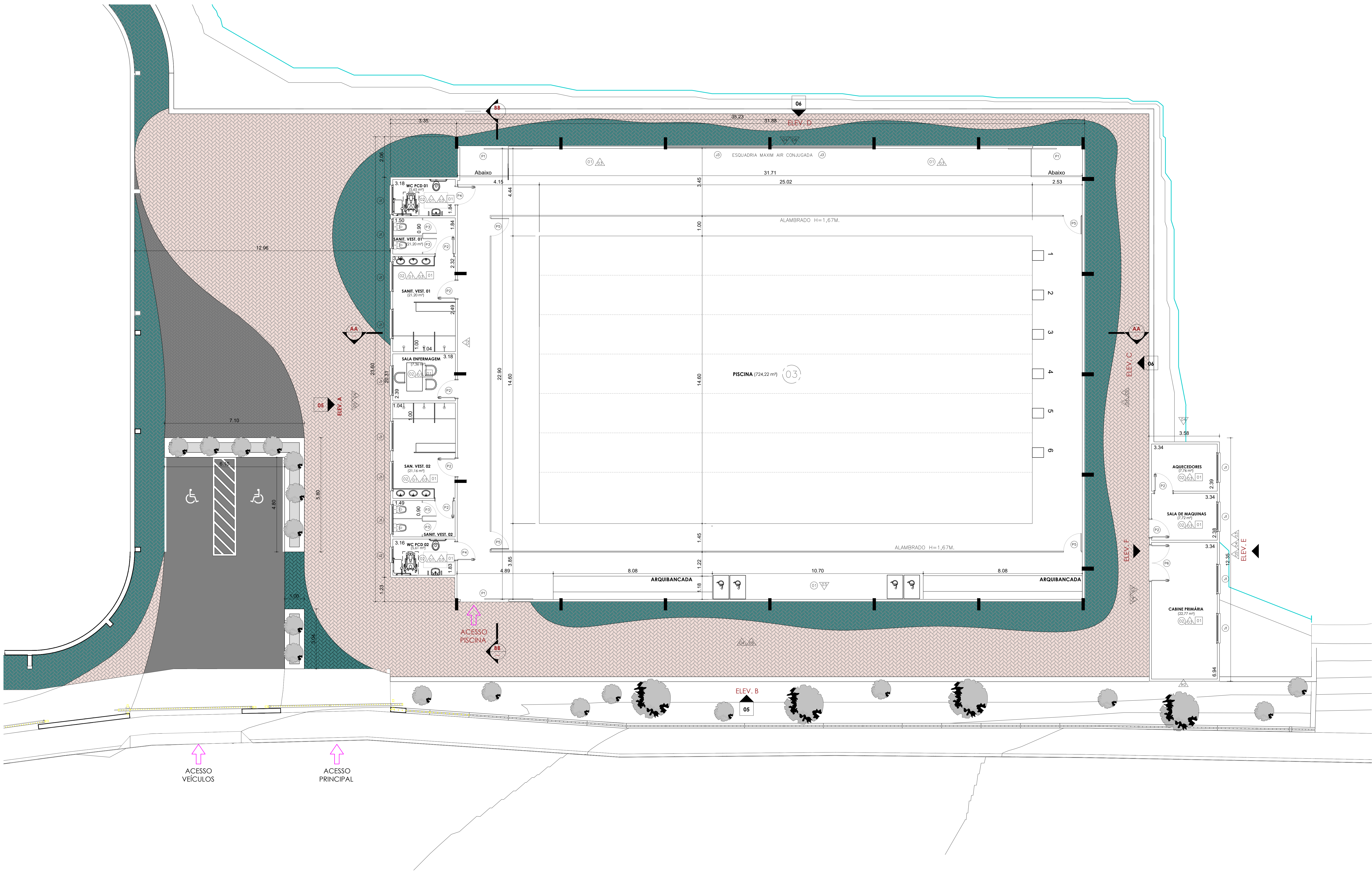
PLANTA PISCINA ESC: 1/75
