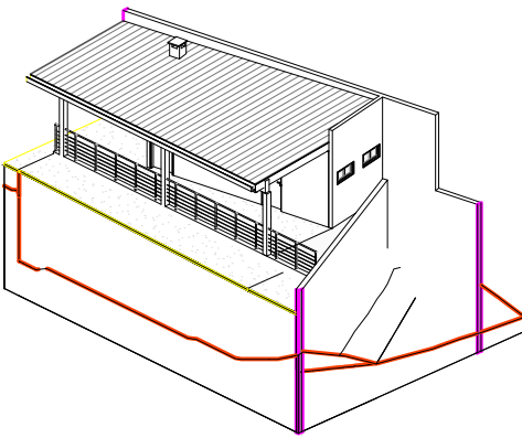
ISOMÉTRICA CHURRASQUEIRA SEM ESC.
