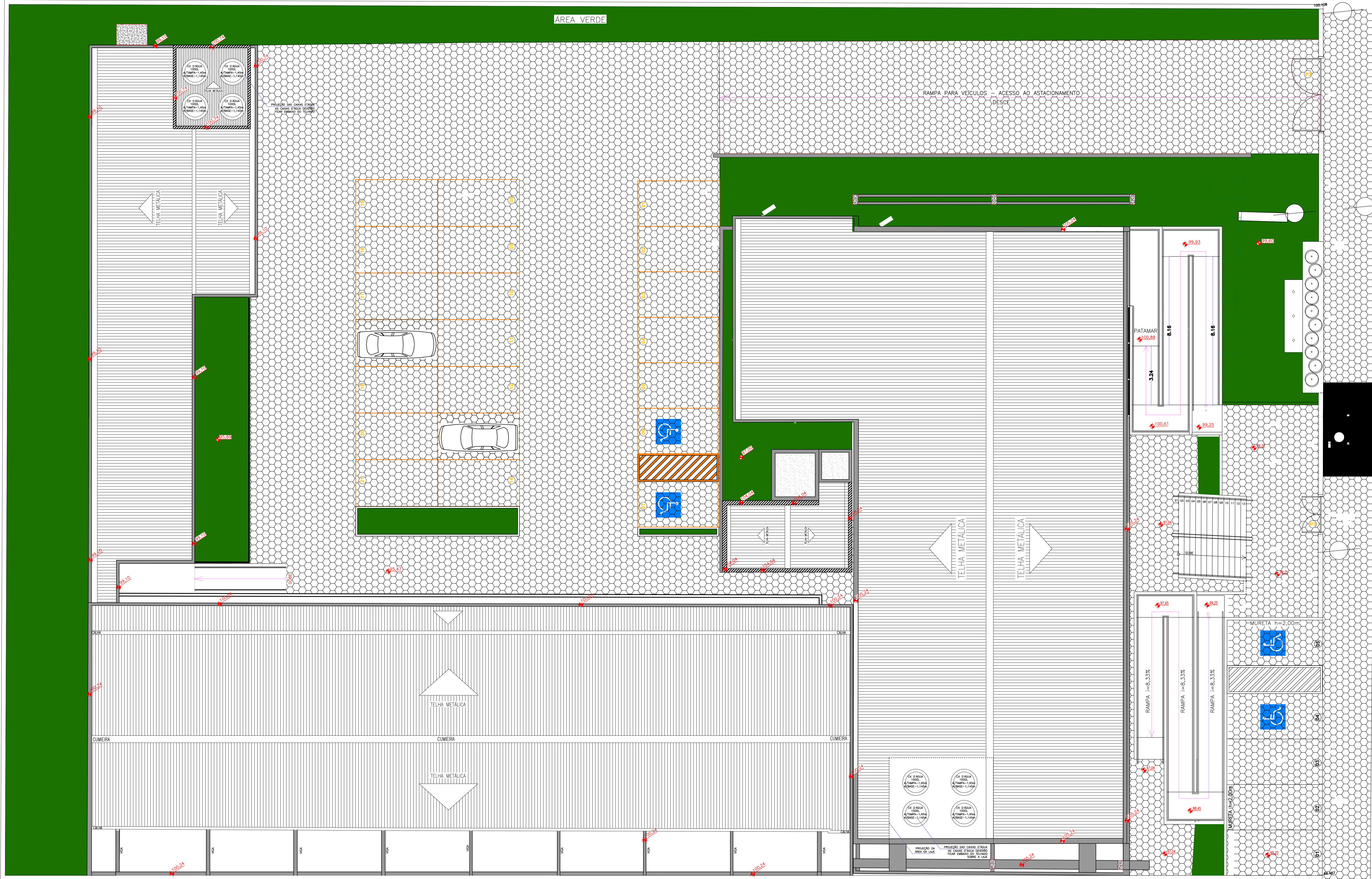
PLANTA COBERTURA escala 1:100
