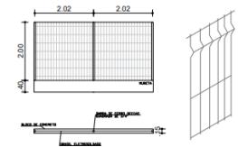
DET. GRADIL ELETROSOLDADO ESC: 1/75
