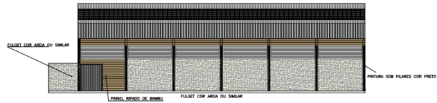
ELEVAÇÃO B ESC: 1/125
