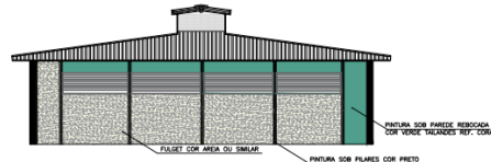
ELEVAÇÃO C ESC: 1/125
