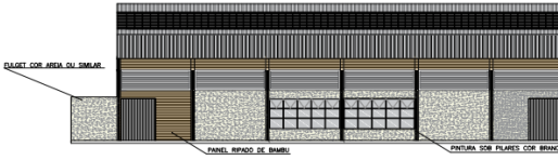
ELEVAÇÃO D ESC: 1/125
