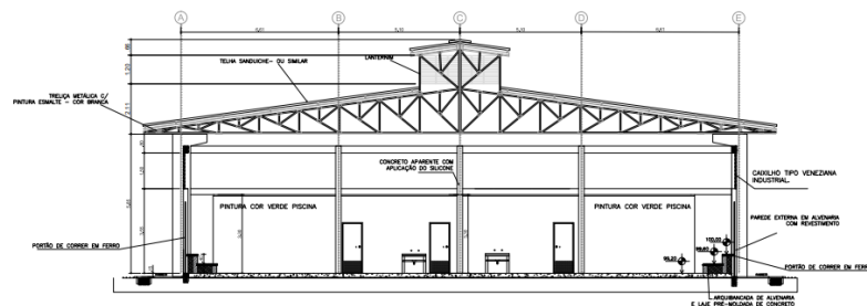
CORTE BB ESC: 1/75
