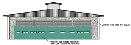
ELEVAÇÃO A ESC: 1/125
