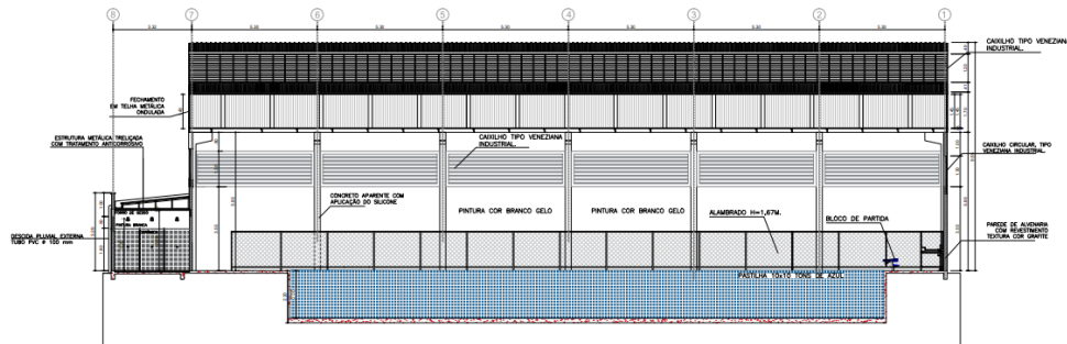
CORTE AA ESC: 1/75
