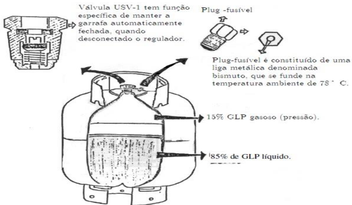
Figura 28 - Estrutura do Botijão P-13
