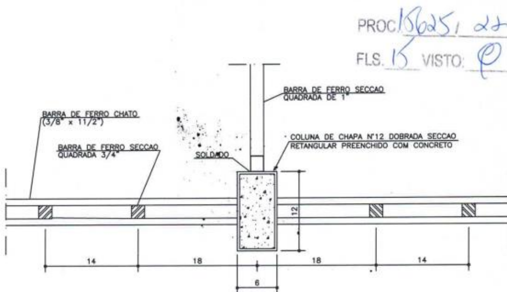
DETALHE 1 ESC. 1:5
