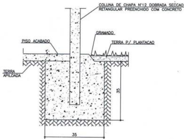
CORTE B-B ESC. 1:10
