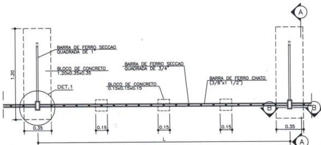
PLANTA ESC. 1:25
