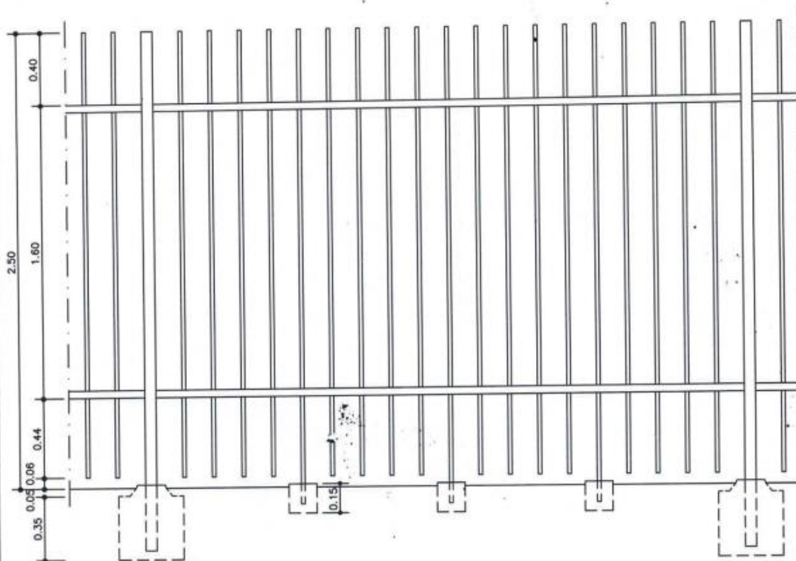
ELEVACAO ESC. 1:25
