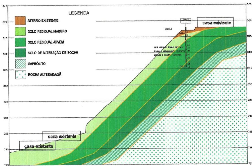
Figura 6 – Perfil Geotécnico B
