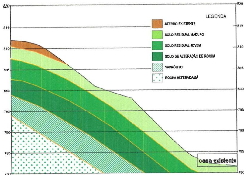
Figura 5 – Perfil Geotécnico A
