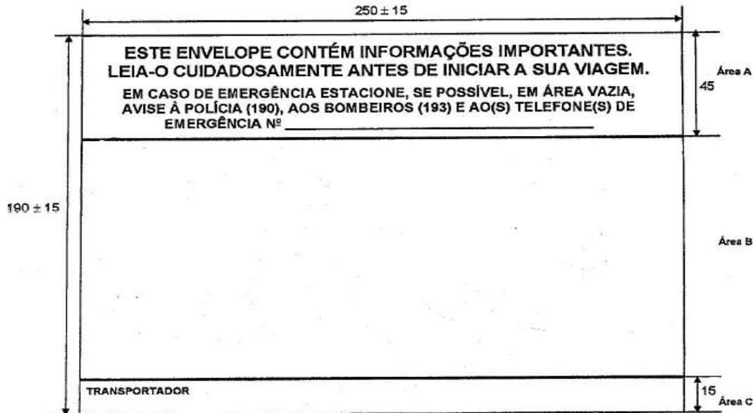
Figura 1 – Dimensões mínimas das áreas A, B e C do envelope (frente)
