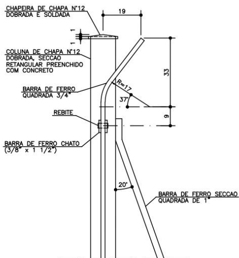
DETALHE 2 ESC. 1:12,5
