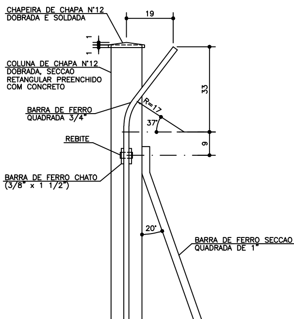
DETALHE 2 ESC. 1:12,5
