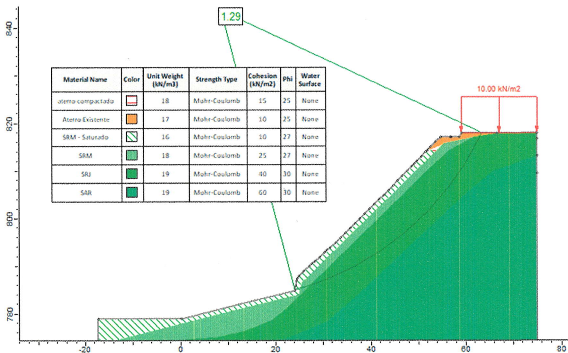
Figura 9 – Saída Gráfica do Perfil Geotécnico B na situação atual, com um fator de segurança de 1,29, considerado INSATISFATÓRIO para condição permanente.
