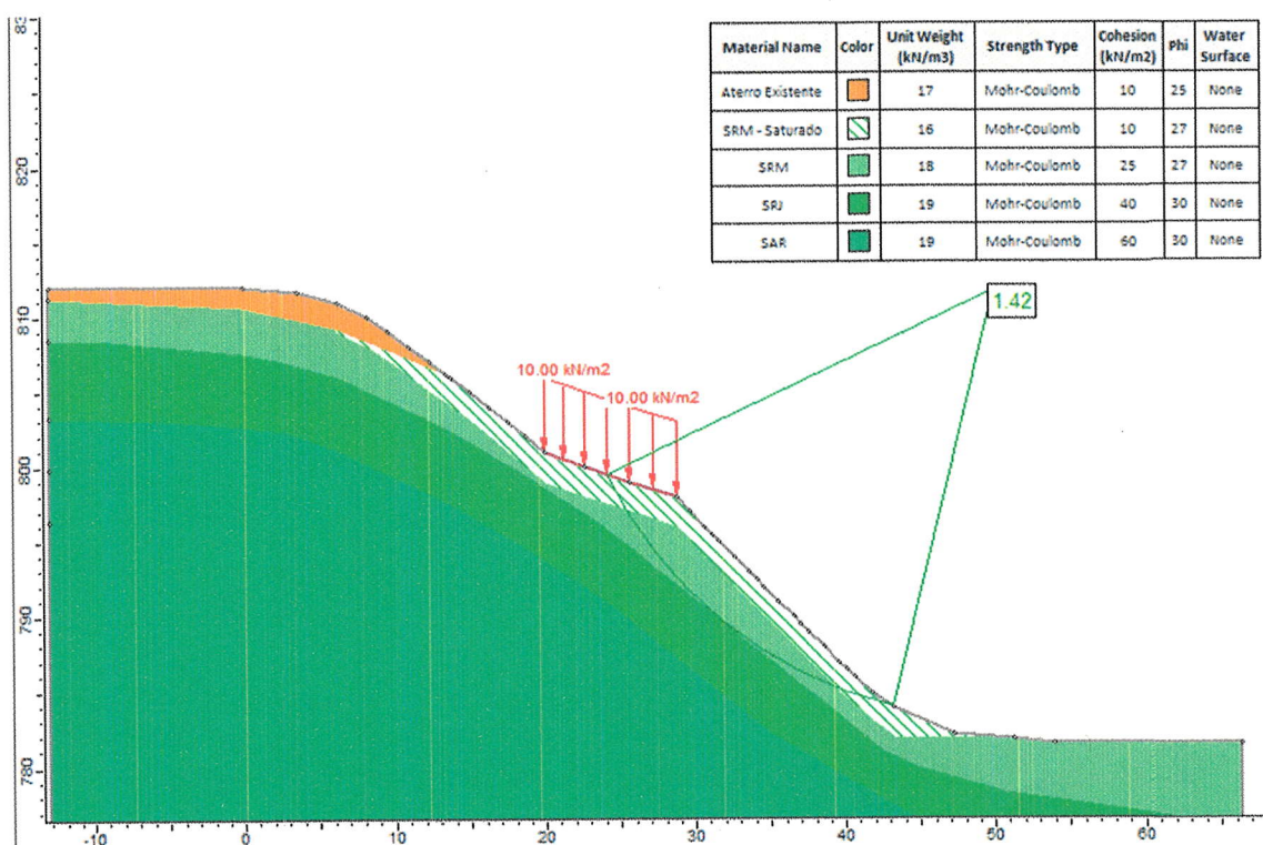
Figura 7 – Saída Gráfica do Perfil Geotécnico A na situação atual, com um fator de segurança de 1,42, considerado INSATISFATÓRIO para condição permanente.
