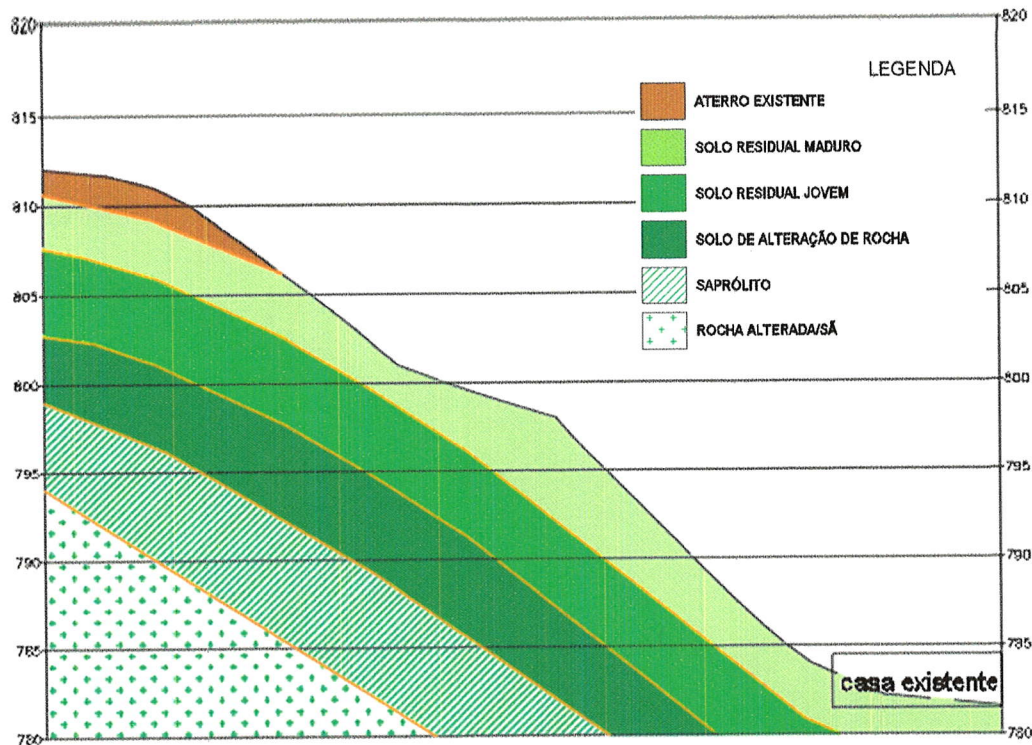
Figura 5 – Perfil Geotécnico A
