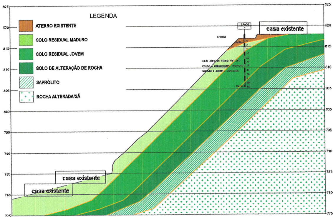
Figura 6 – Perfil Geotécnico B
