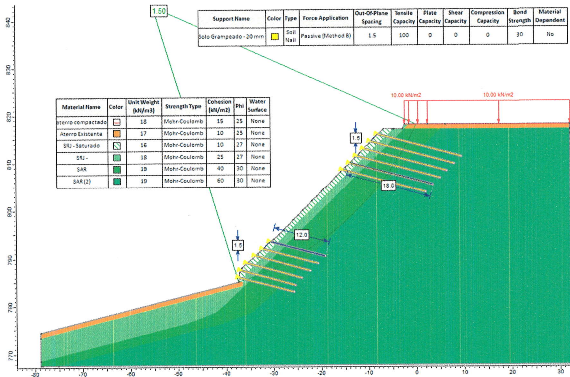
Figura 11 – Saída Gráfica do Perfil Geotécnico B, com um fator de segurança de 1,50, considerado SATISFATÓRIO para condição permanente.
