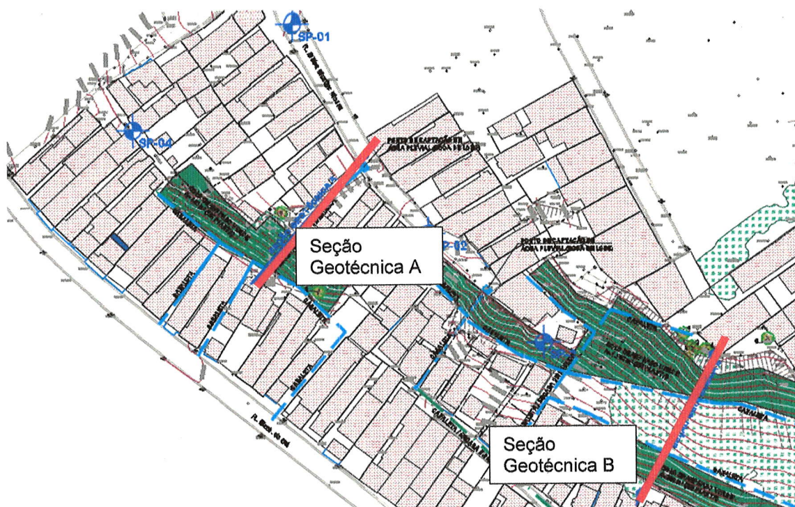
Figura 4 – Locais das seções típicas analisadas – Seção A e Seção B.
