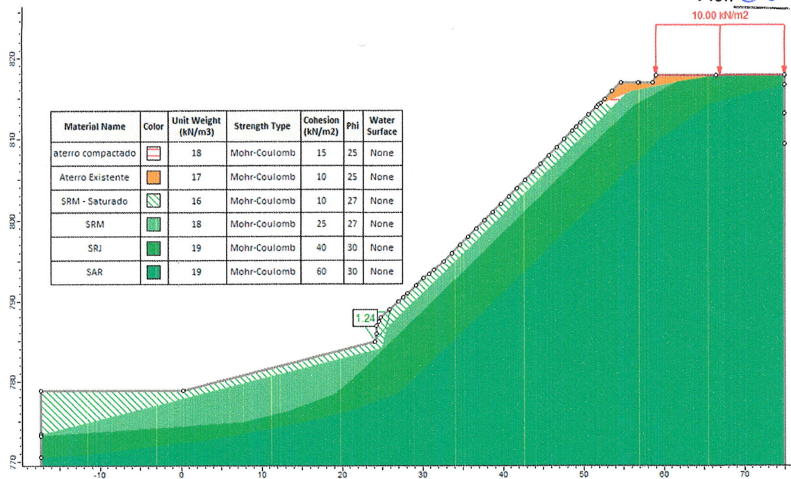
Figura 8 – Saída Gráfica do Perfil Geotécnico B na situação atual, com um fator de segurança de 1,24 (no pé do talude), considerado INSATISFATÓRIO para condição permanente.
