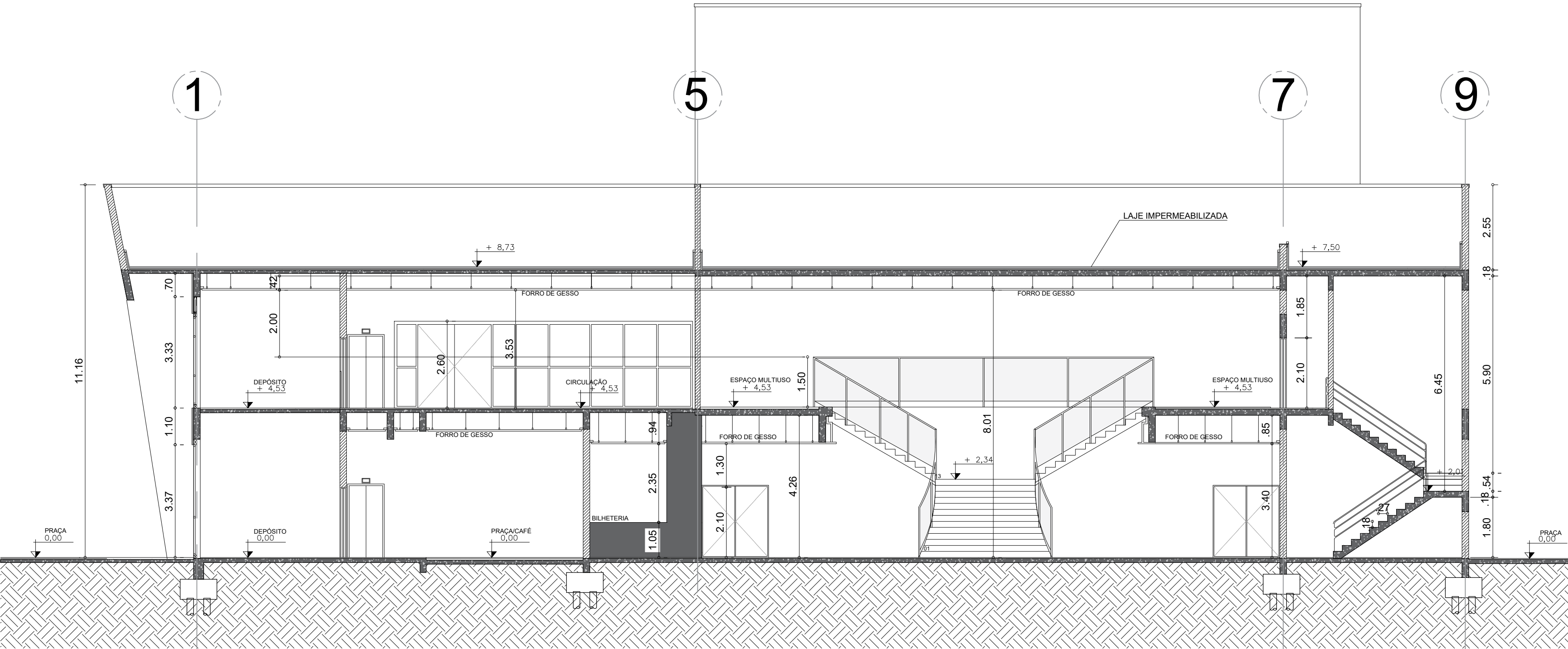
CORTE BB ESC: 1/100
