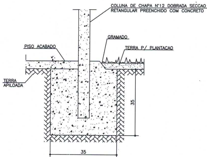
CORTE B-B ESC. 1:10
