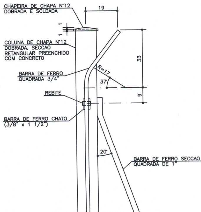
DETALHE 2 ESC. 1:12,5
