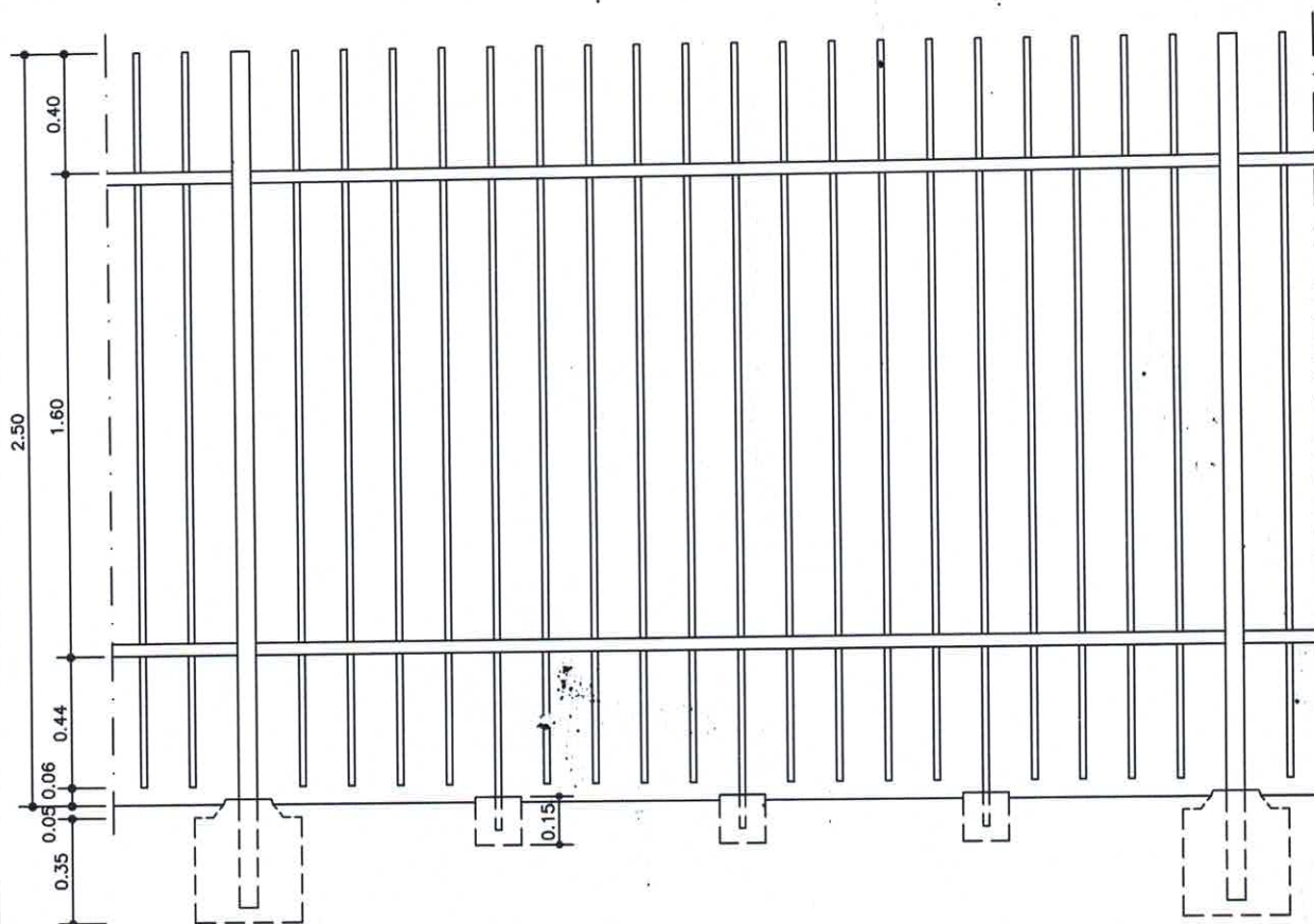
ELEVACAO ESC. 1:25
