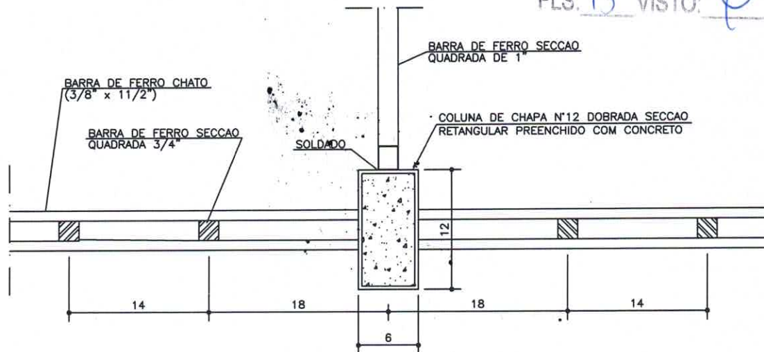
DETALHE 1 ESC. 1:5
