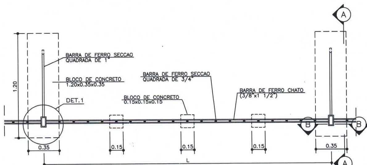
PLANTA ESC. 1:25
