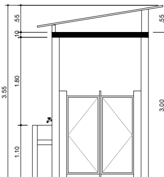
CORTE AA VESTIÁRIO ESC: 1/100
