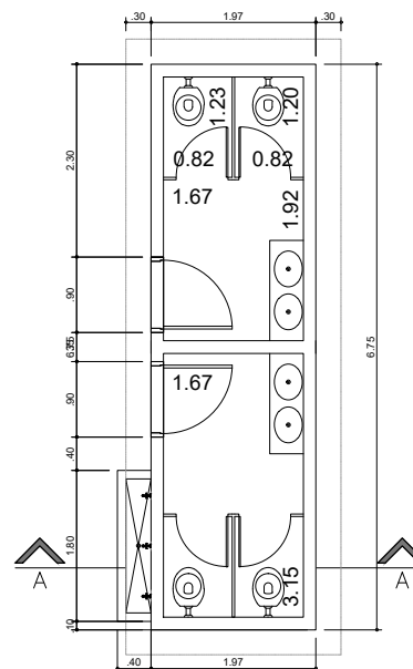
AMPLIAÇÃO VESTIÁRIO ESC: 1/100
