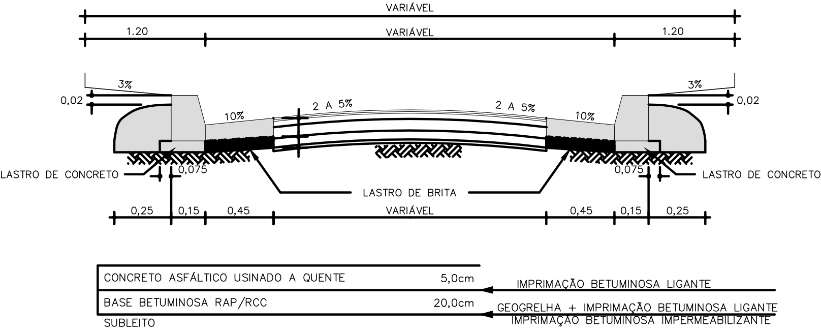
SEÇÃO REFORÇO DE PAVIMENTO SEM ESCALA
