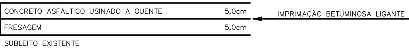
SEÇÃO TÍPICA RECAPEAMENTO ASFÁLTICO SEM ESCALA
