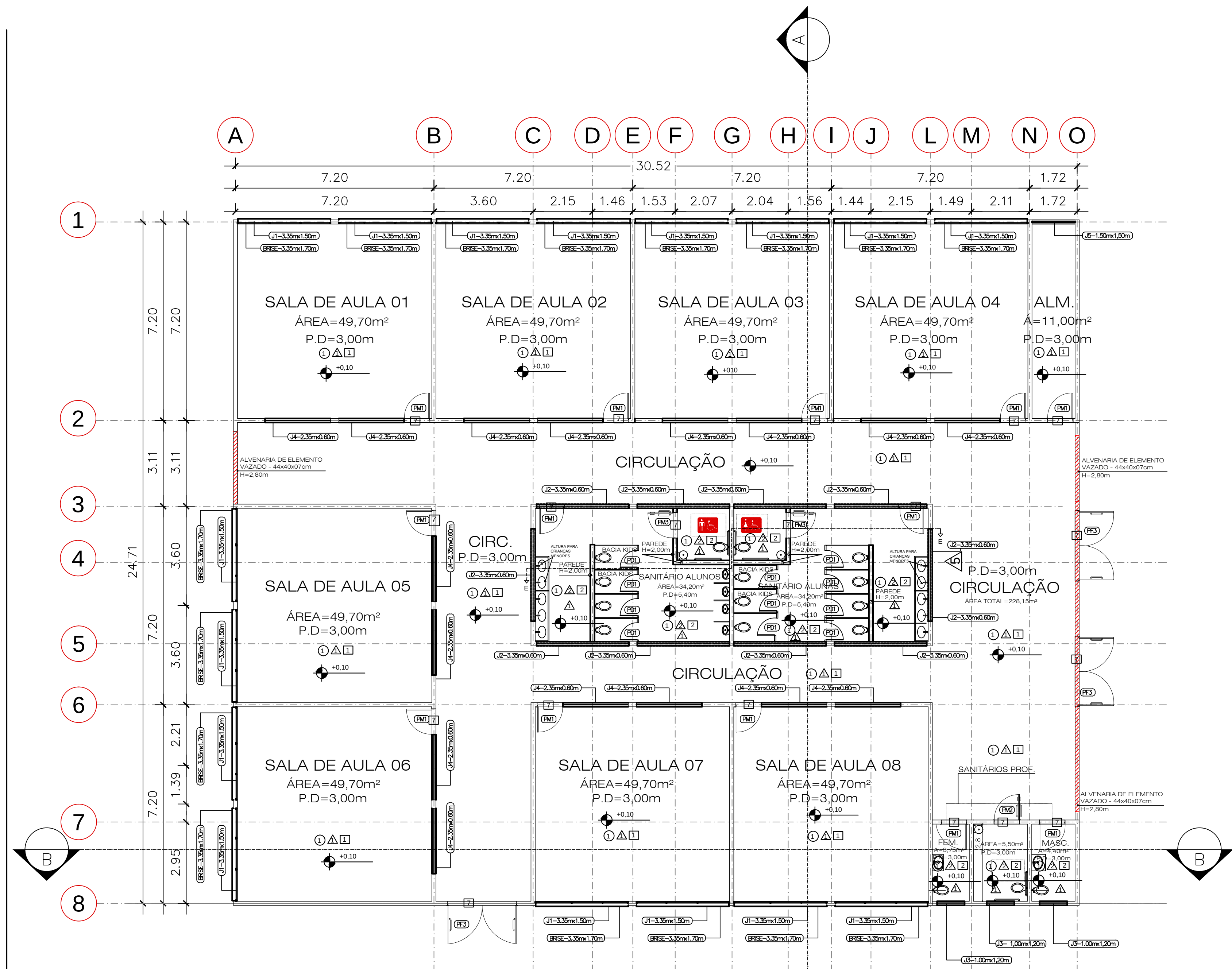
PLANTA – TÉRREO ESCALA 1:100
