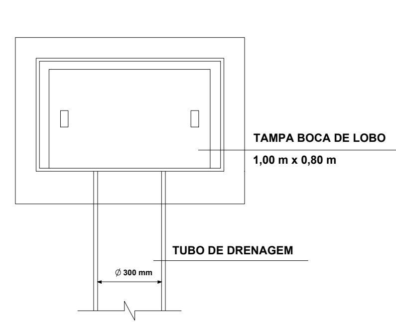
DETA LHAMENTO BOCA DE LOBO SIMPLES:
