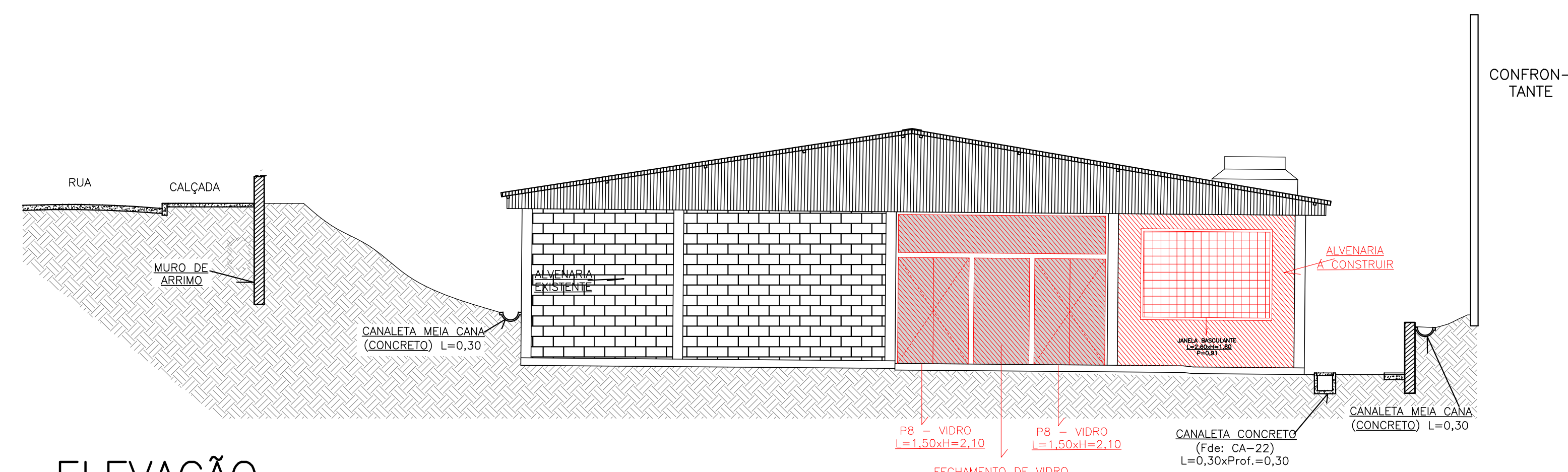
ELEVAÇÃO POSTERIOR ESCALA 1:75
