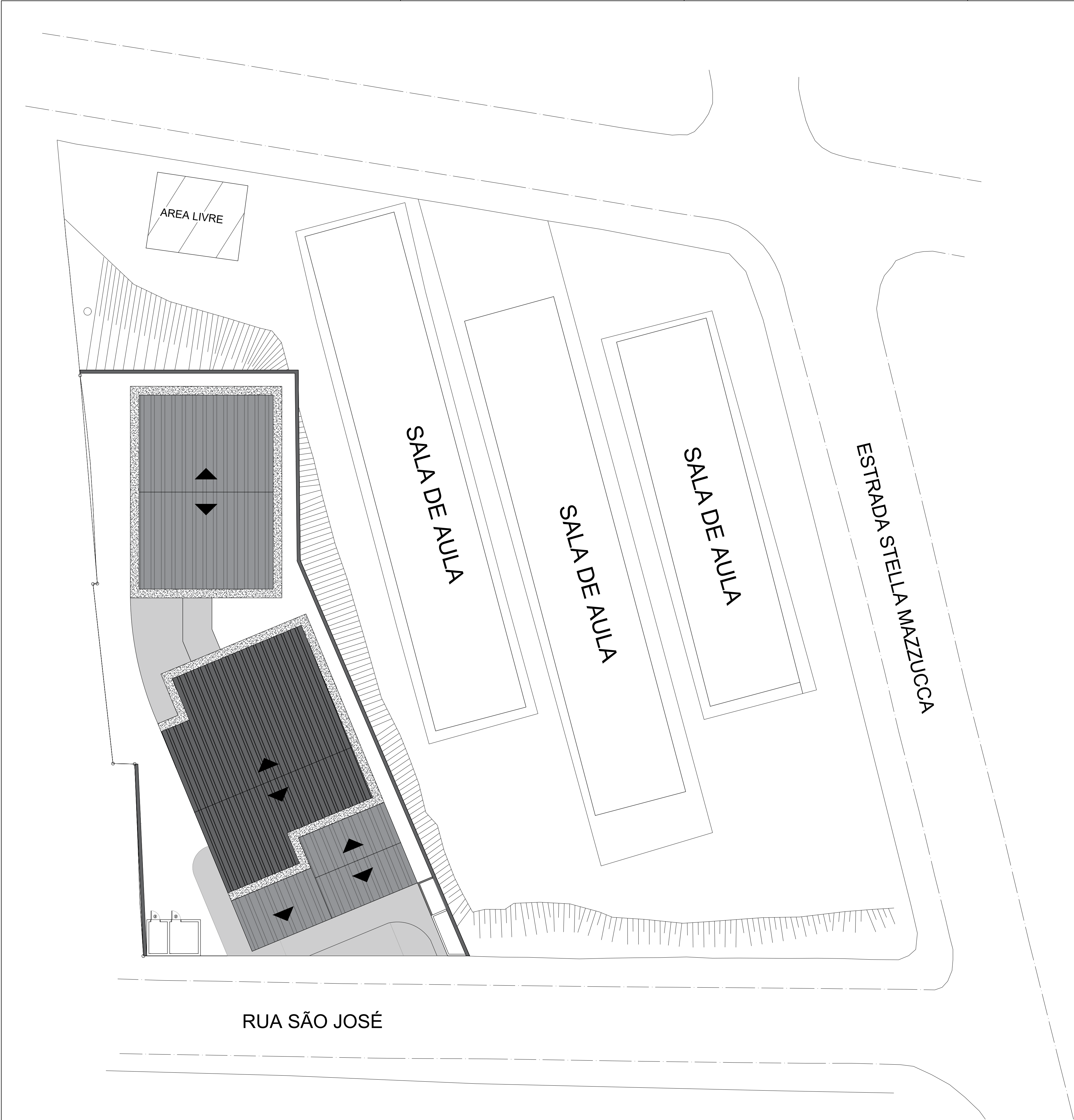
PLANTA DE IMPLANTAÇÃO COM COBERTURA ESC: 1/200
