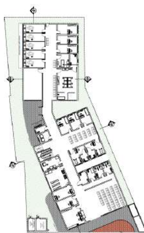
PLANTA DE LAYOUT ARQUITETURA TÉRREO ESC: 1/200
