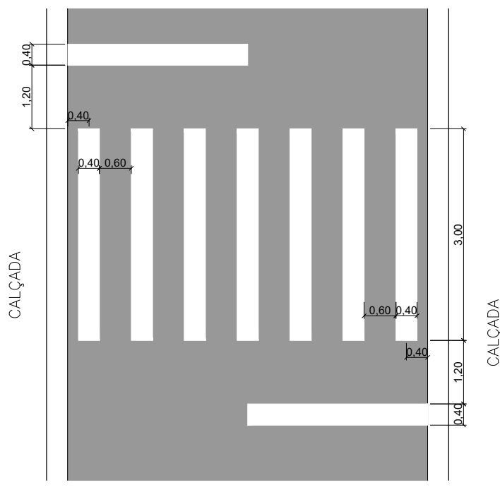
DETALHE DE FAIXA DE PEDESTRE E FAIXA DE RETENÇÃO S/ ESC.
