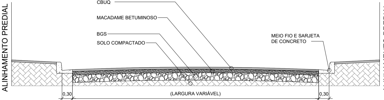
SEÇÃO-TIPO DE PAVIMENTAÇÃO S/ ESC.
