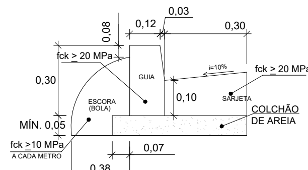
DETALHE DE GUIA E SARJETA ESCALA 1:25
