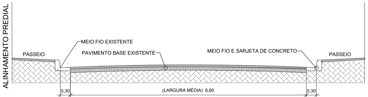
SEÇÃO-TIPO DE RECAPEAMENTO S/ ESC.
