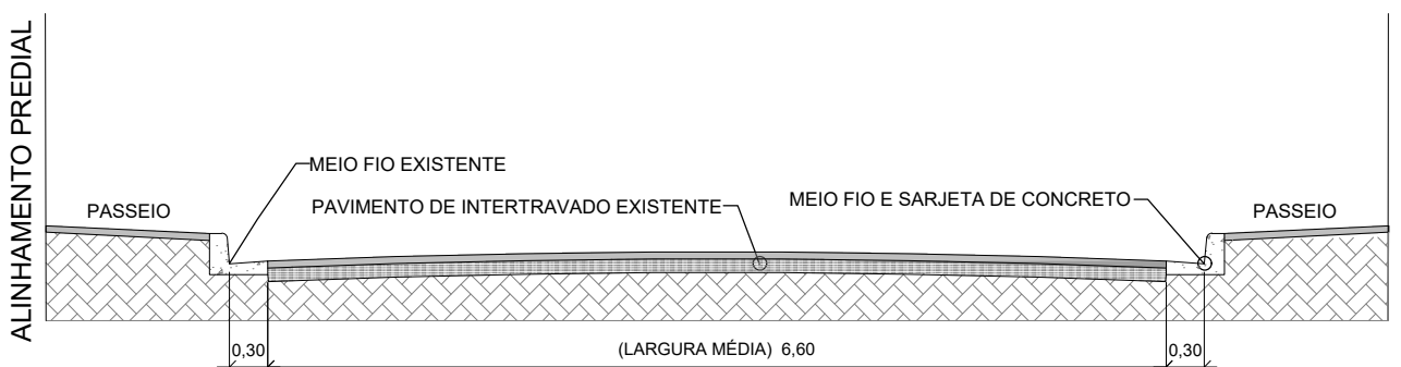
SEÇÃO-TIPO DE CAPEAMENTO ASFÁLTICO SOBRE INTERTRAVADO S/ ESC.
