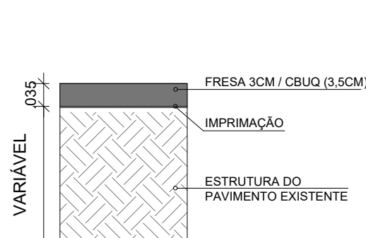
DETALHE TÍPICO DE FRESA E RECAPE ESCALA 1:25
