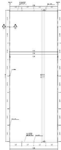
PLANTA DE FUNDAÇÃO QUADRA DE AREIA ESC: 1/125
