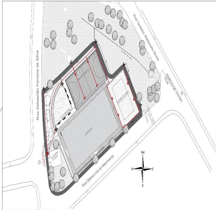
PLANTA DE DISTRIBUIÇÃO ELÉTRICA ESC: 1/400
