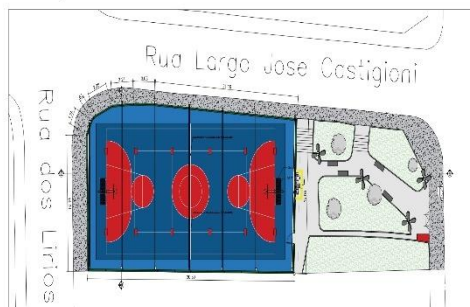
PLANTA IMPLANTAÇÃO QUADRA DE ESPORTES ESC: 1/233
