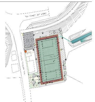
PLANTA DE IMPLANTAÇÃO Escala: 1/50
