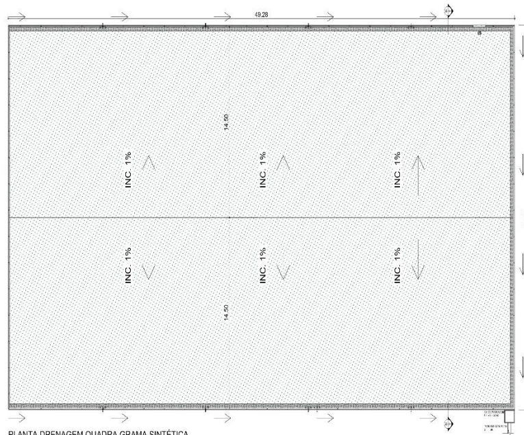
PLANTA DRENAGEM QUADRA GRAMA SINTÉTICA ESC: 1/100
