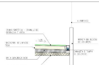
AMPLIAÇÃO CANALETA ESC: 1/100
