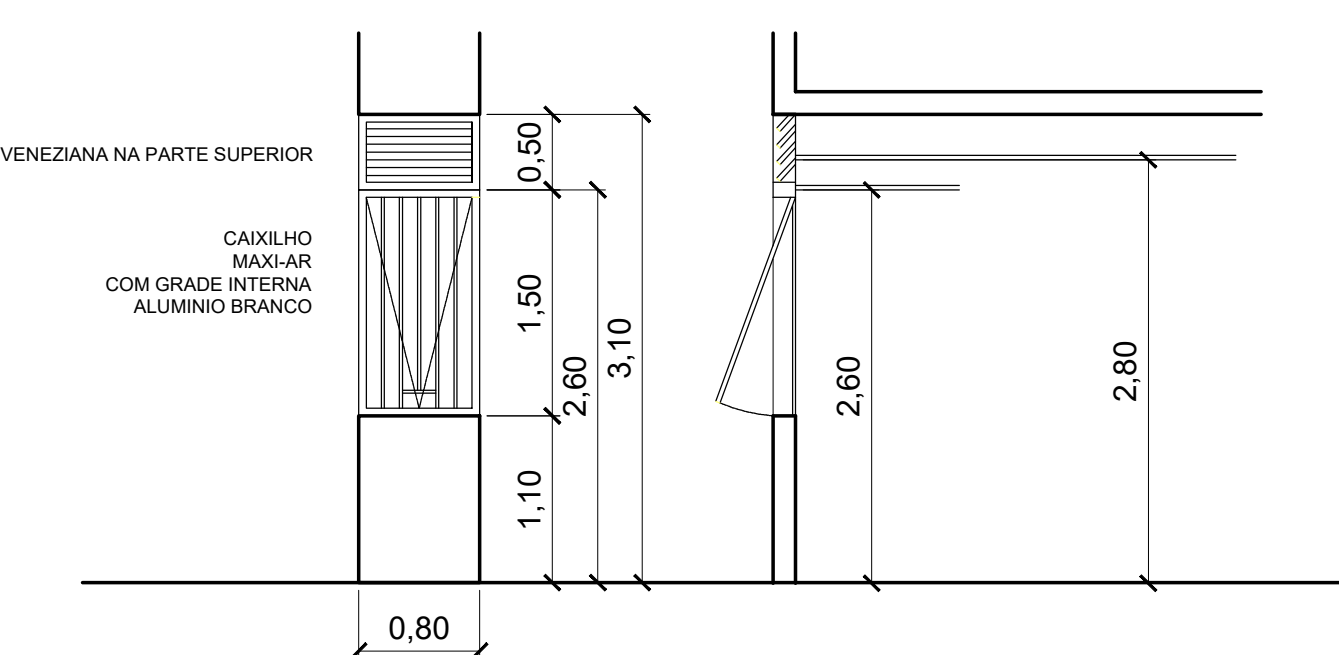
CAIXILHO SALAS ESCALA 1:50
