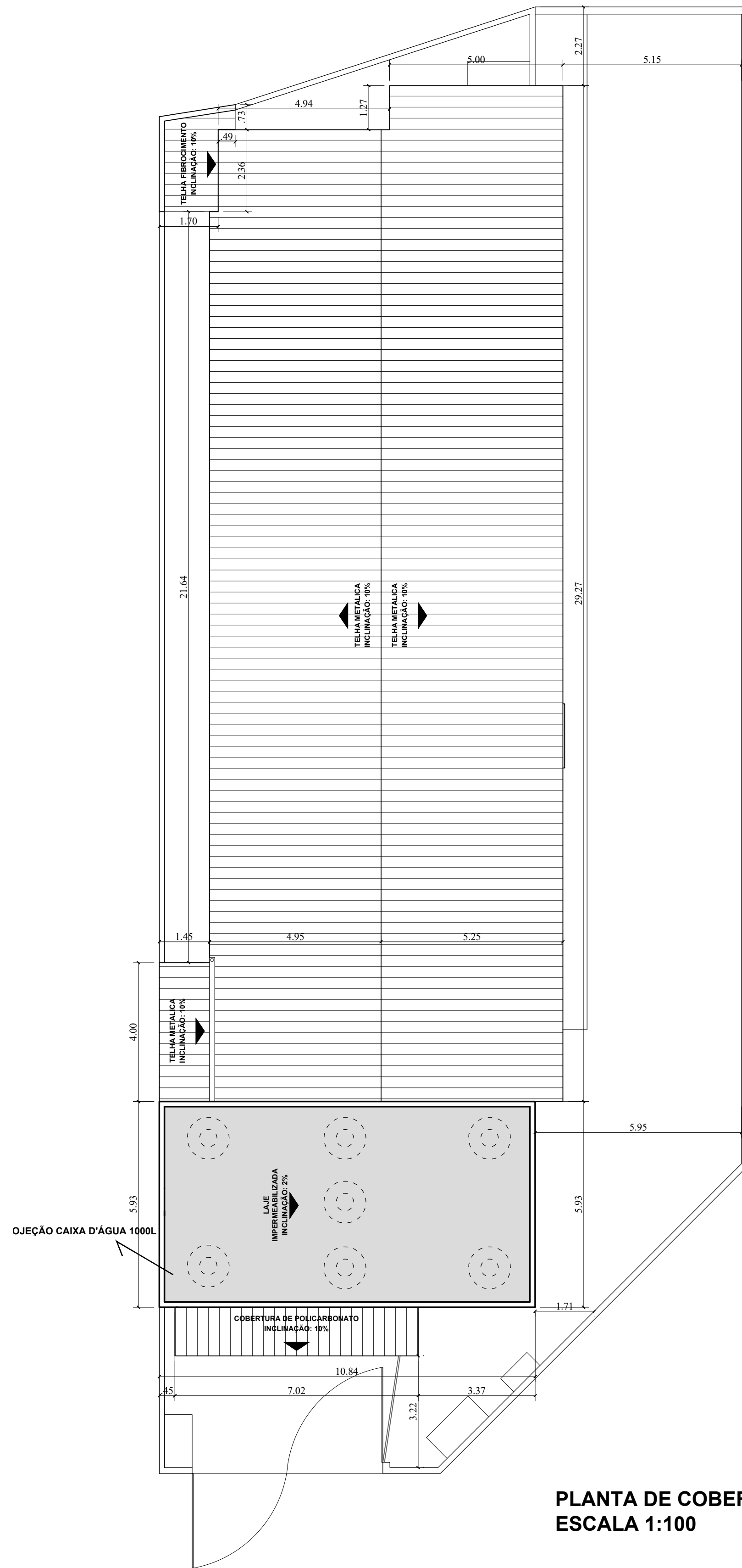
PLANTA DA PROPOSTA ESCALA 1:100
