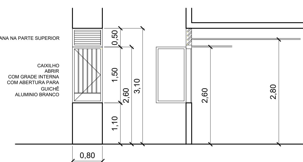
CAIXILH FARMÁC ESCALA 1:80
