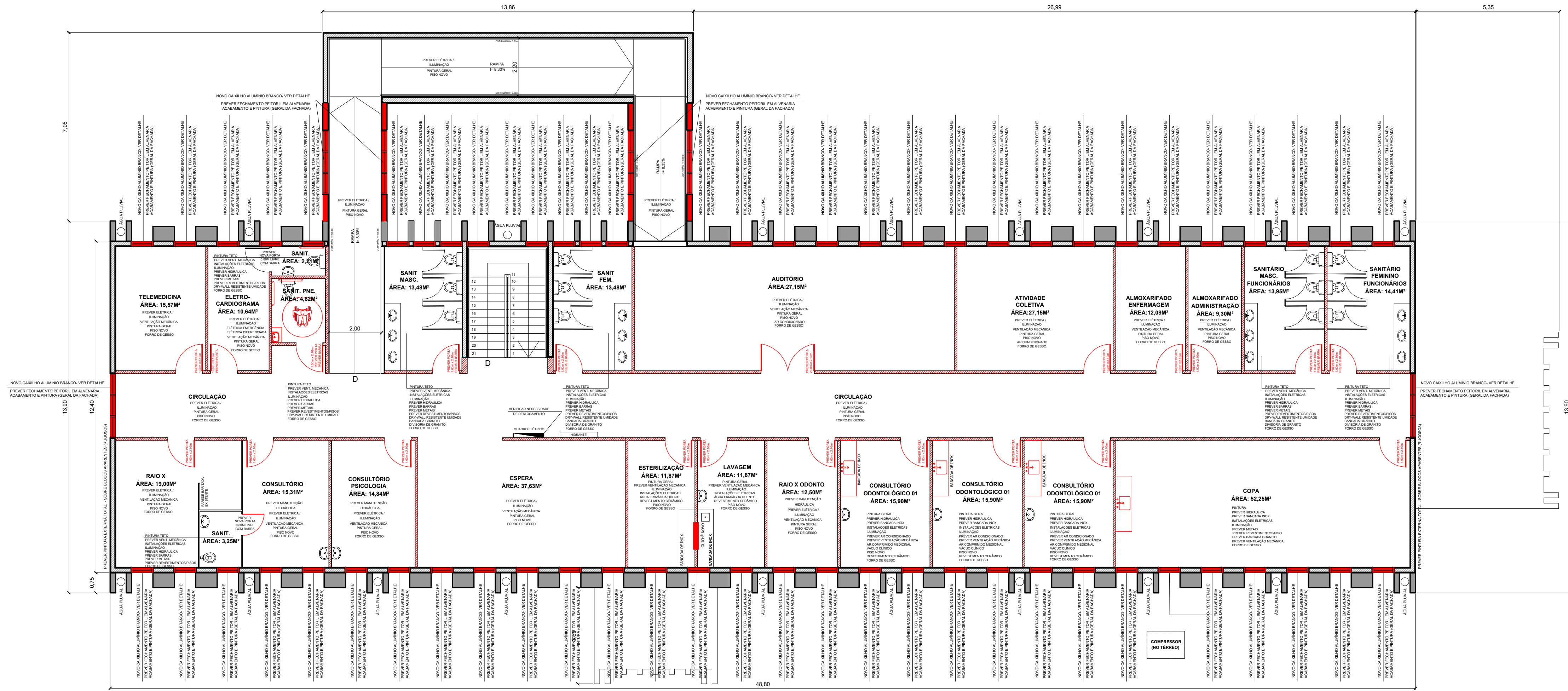
Pav. Superior Escala 1:100
