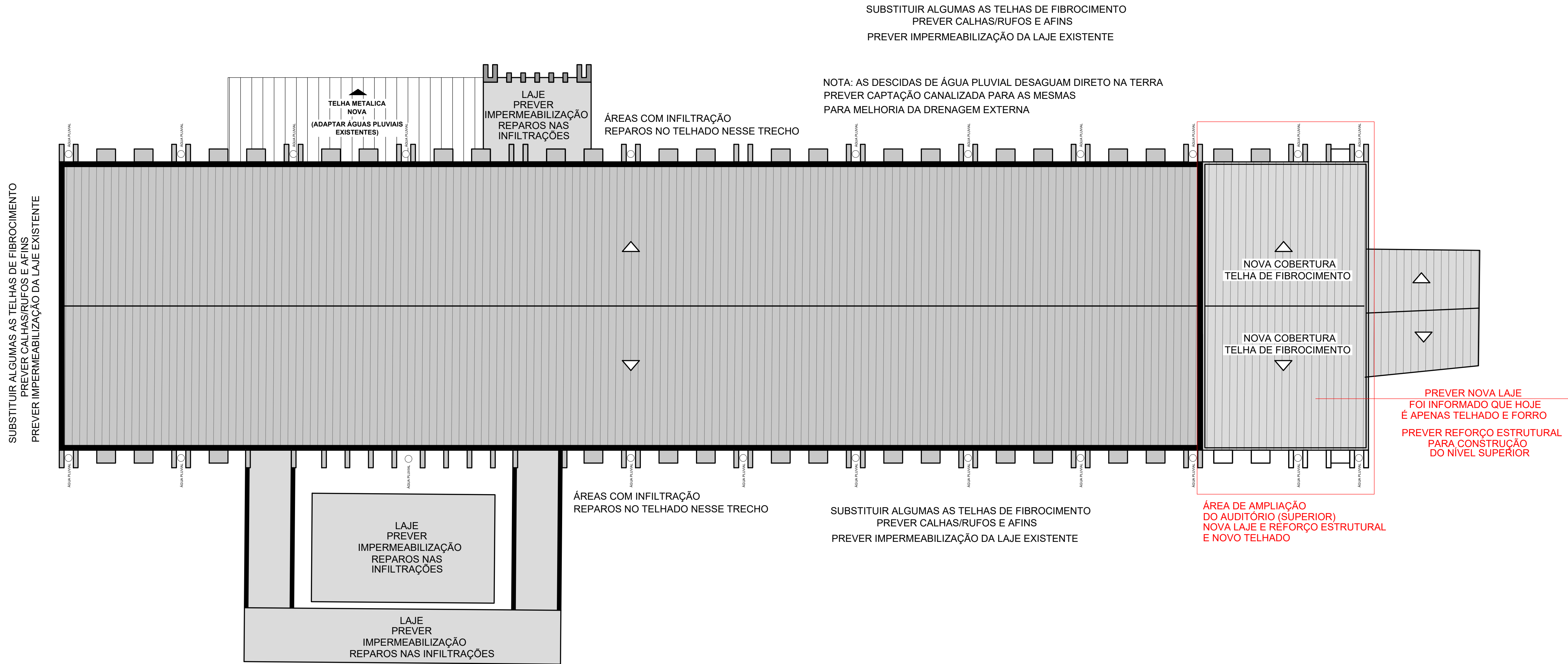
PLANTA DE COBERTURA Escala 1:100
