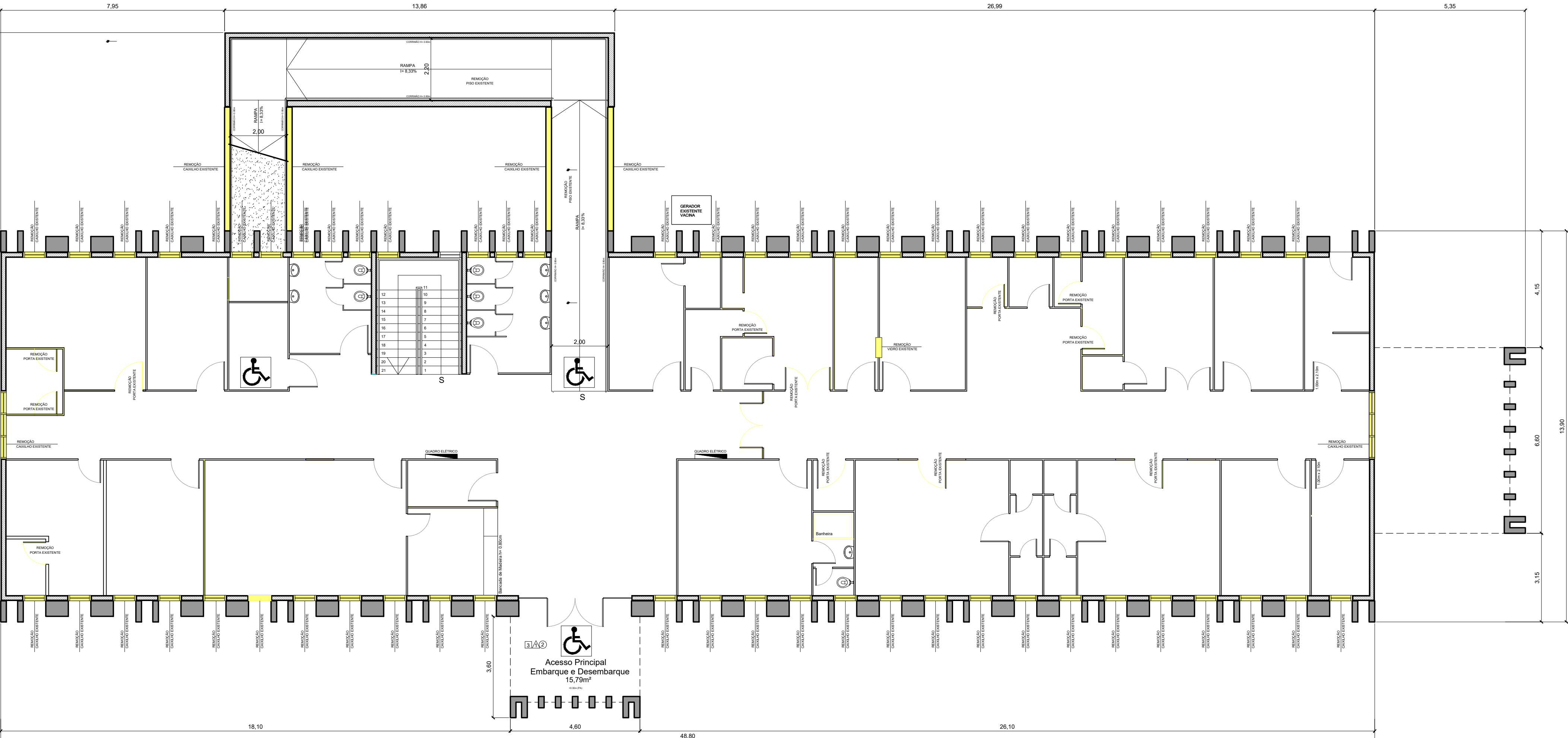
Pav. Térreo Escala 1:100
