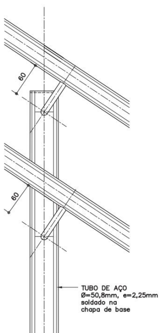
DET. 5 ESC. 1:5 MEDIDAS EM MILÍMETROS
