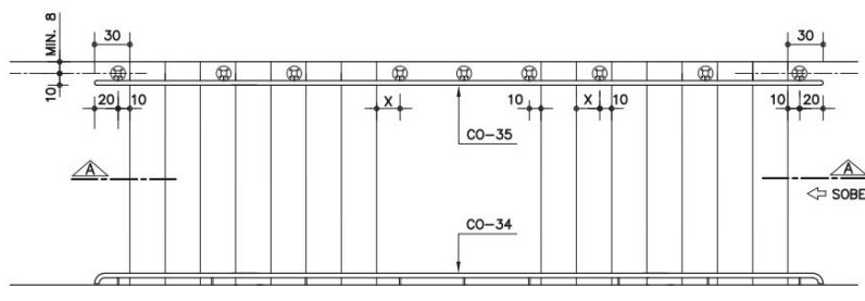
PLANTA GENÉRICA DE ESCADA ESC. 1:50
