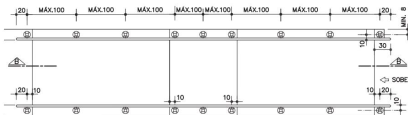
PLANTA GENÉRICA DE RAMPA ESC. 1:50
