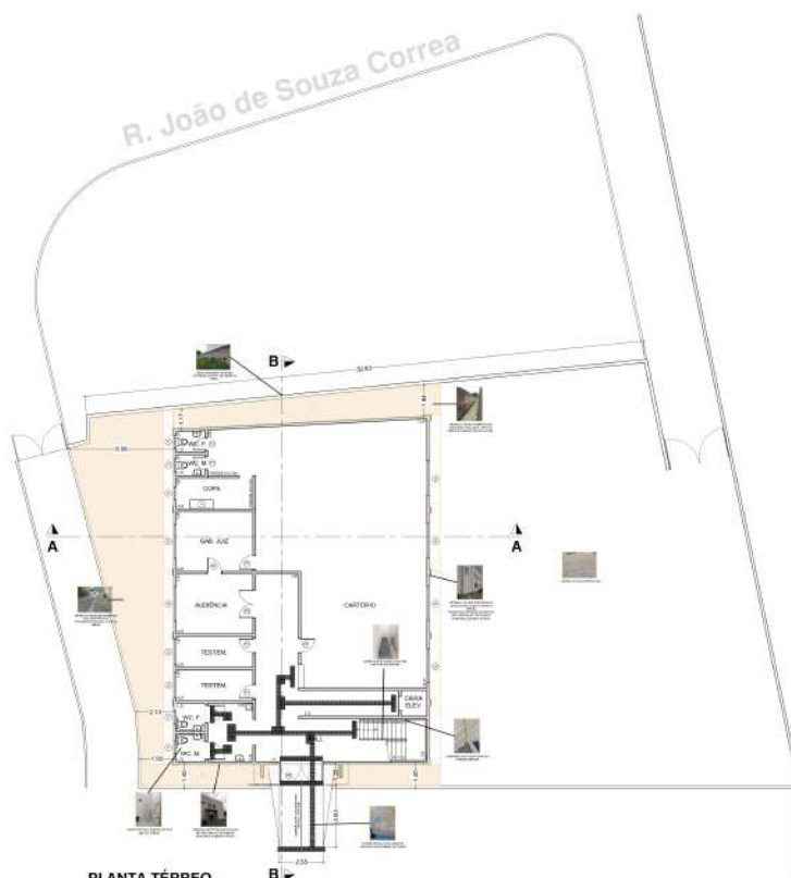
PLANTA TÉRREO
